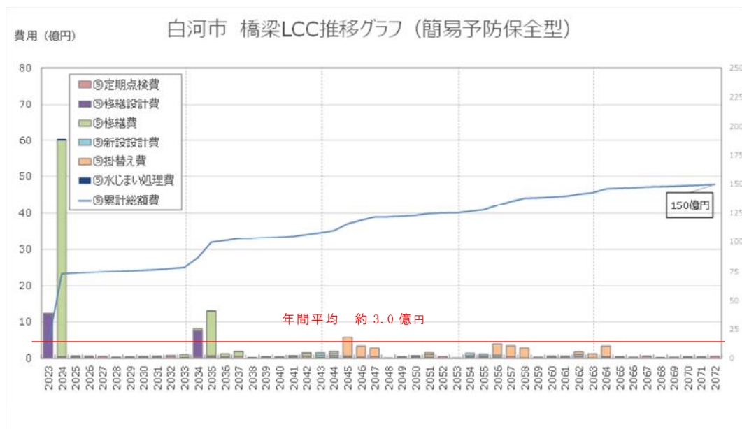
図 9.3 簡易予防保全型の維持管理コスト
