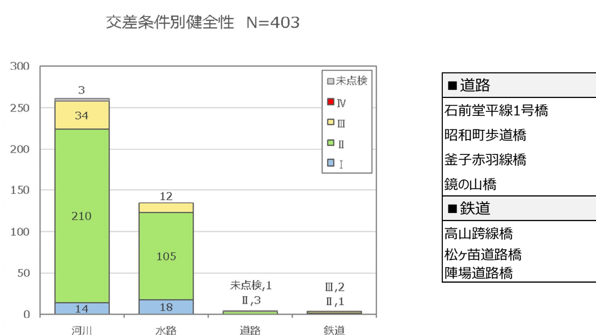
図 2.27 交差条件別橋梁の健全性
