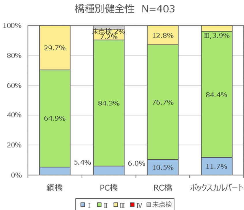
図 2.22 橋種別にみた橋梁の健全性割合
