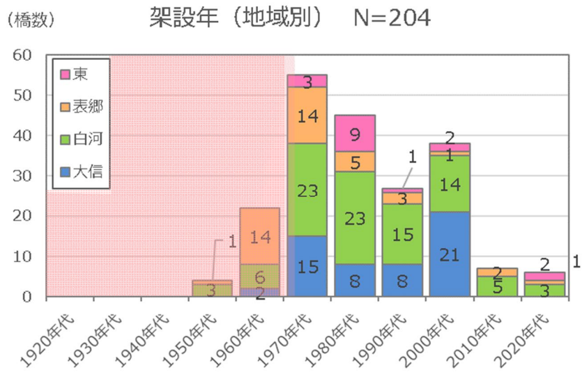
図 2.6 地域区別の架設年別橋梁数
