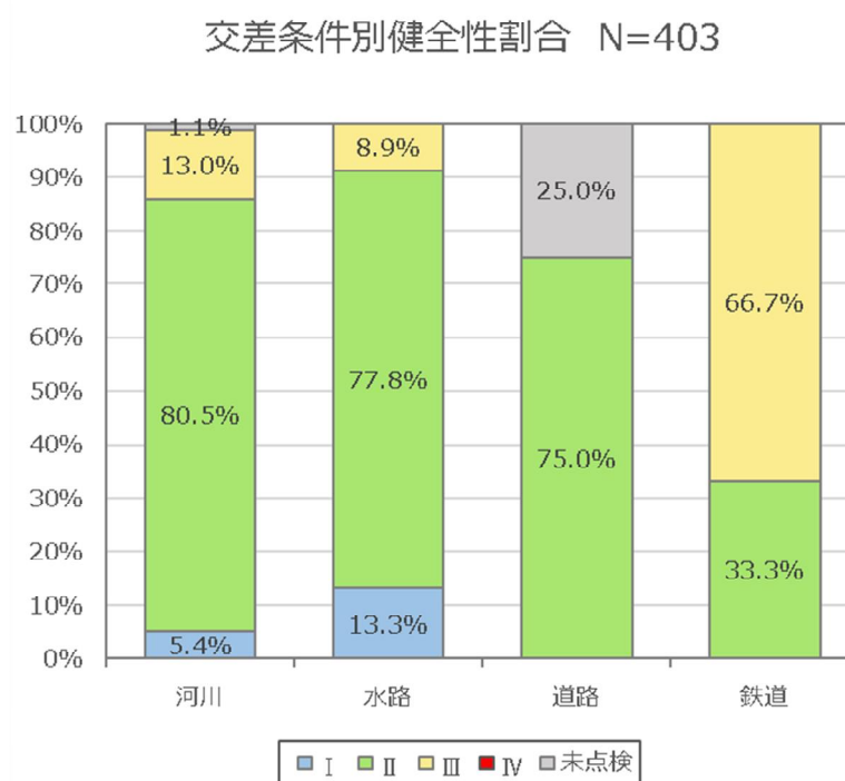
図 2.28 交差条件別橋梁の健全性
