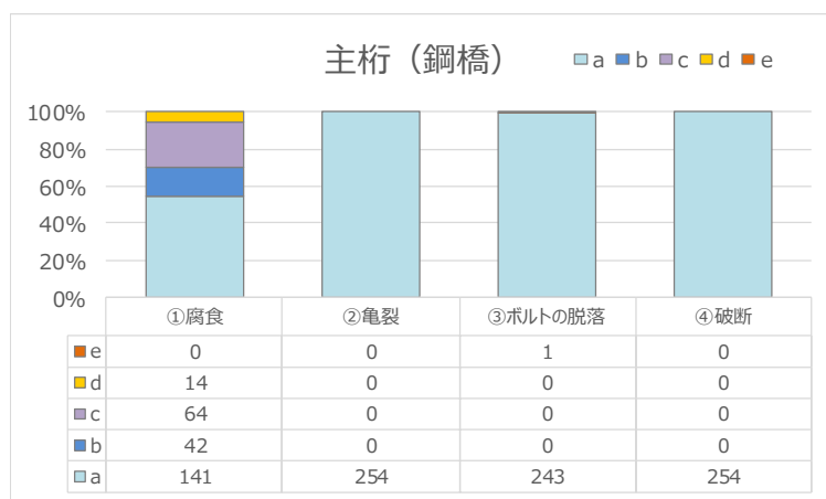
図 4.13 主桁（鋼橋）の損傷数とその程度割合
