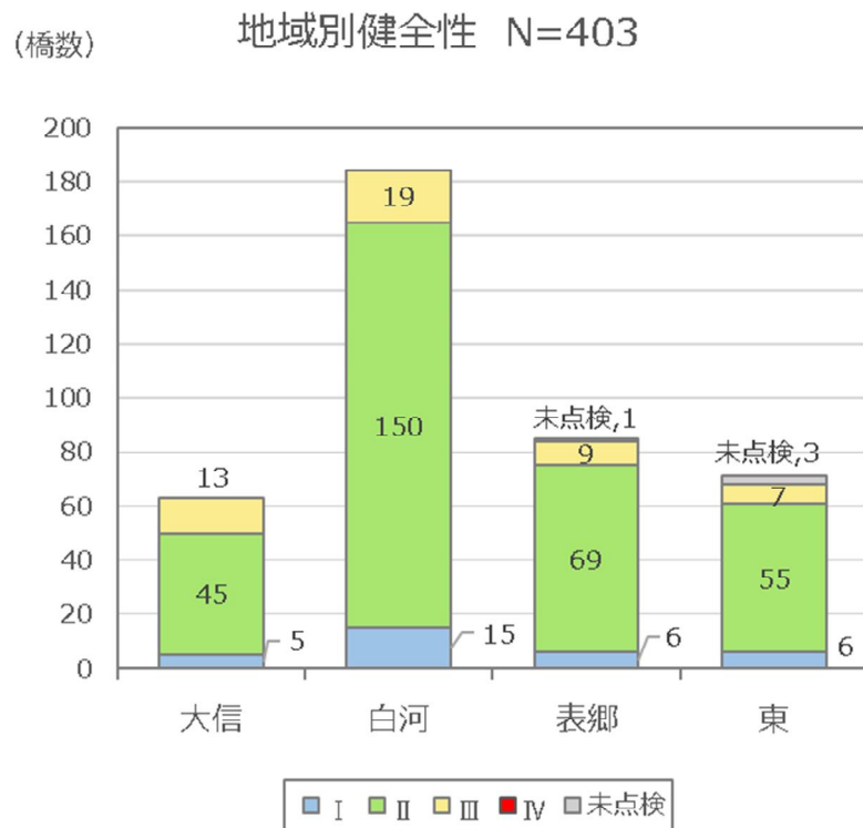
図 2.18 地域別にみた橋梁の健全性
