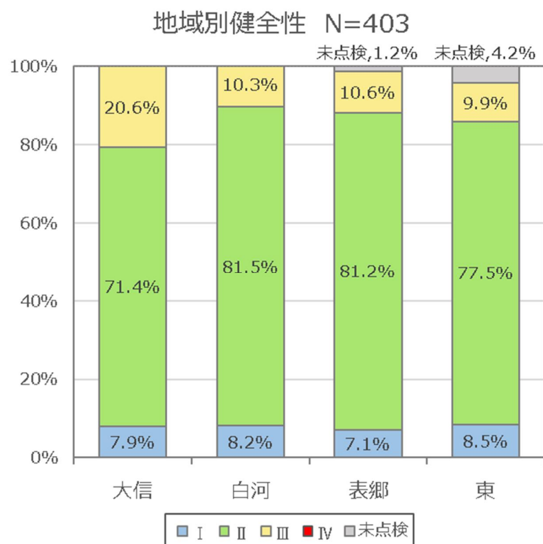
図 2.19 地域別にみた橋梁の健全性割合
