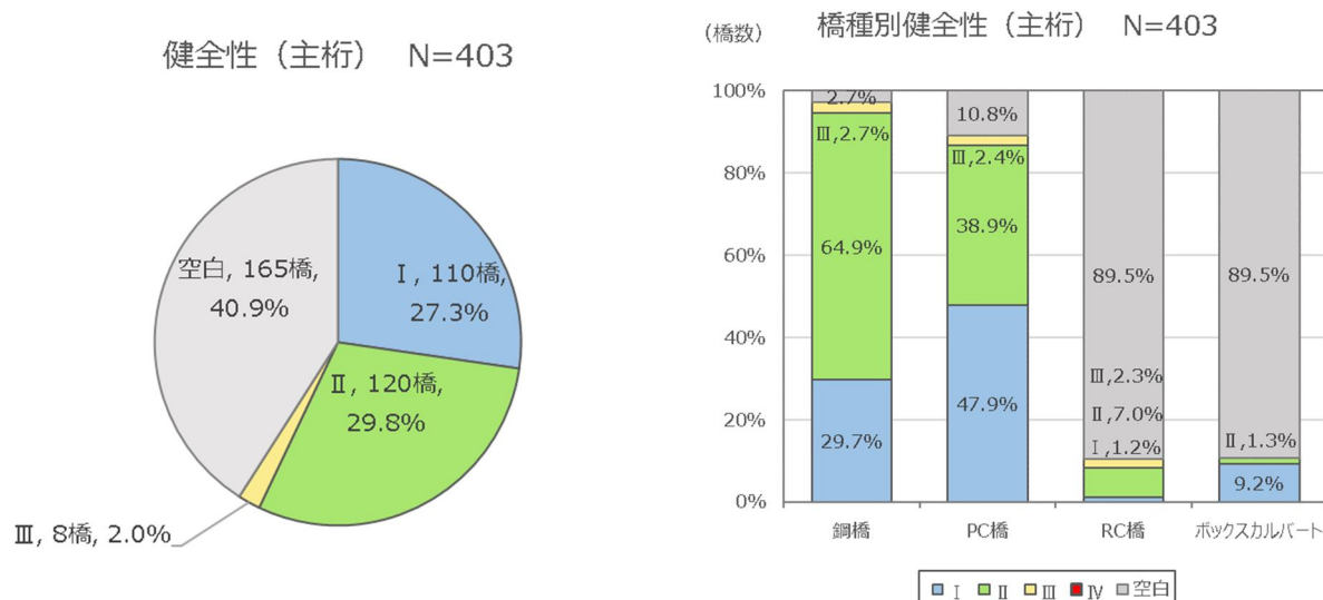
図 2.29 主桁の健全性分布（左：健全性の割合、右：橋種別の健全性）
