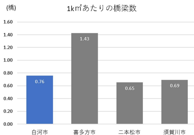
図 4.5 1k㎡あたりの橋梁数
