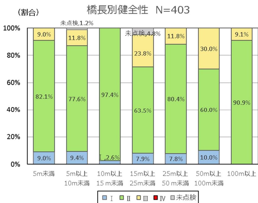
図 2.26 橋長別橋梁の健全性
