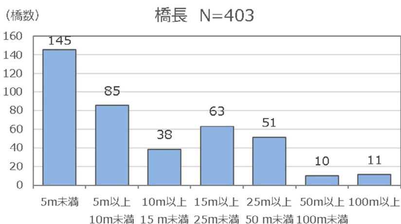
図 2.8 橋長別の橋梁数
