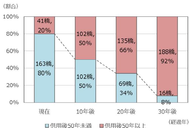
図 2.5 供用後 50 年以上経過した橋梁の割合推移
