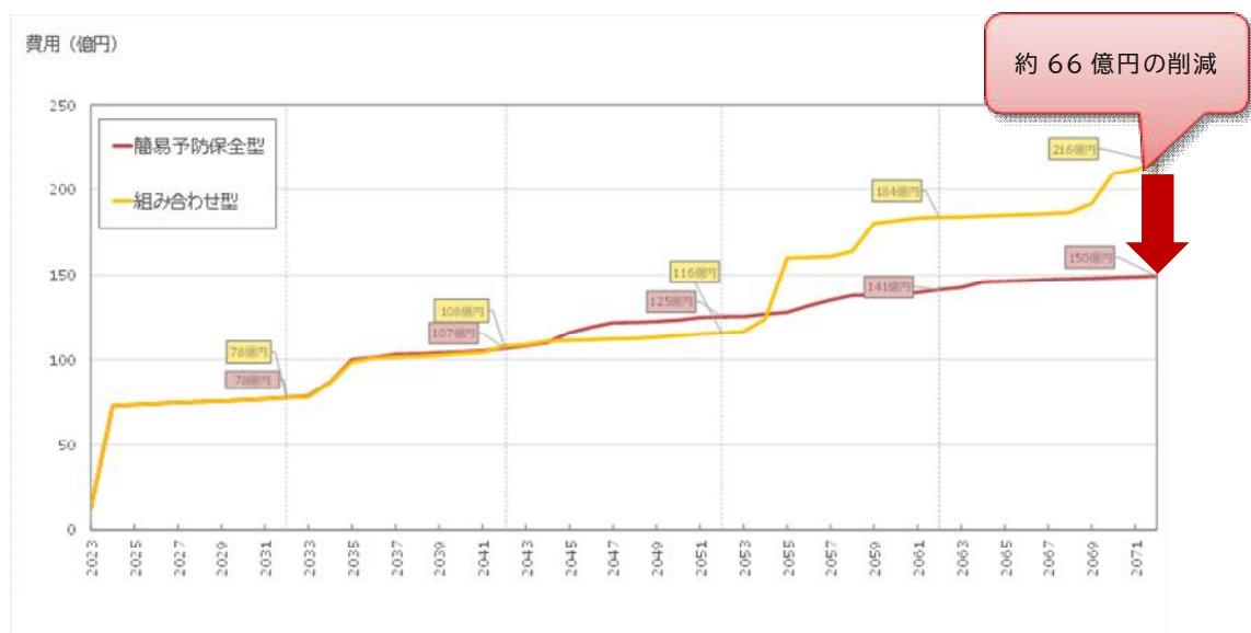
図 9.4 組み合わせ型と簡易予防保全型の累計維持管理コスト
