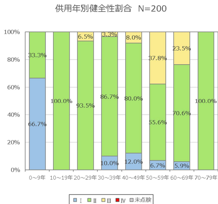
図 2.24 供用年別にみた橋梁の健全性割合
