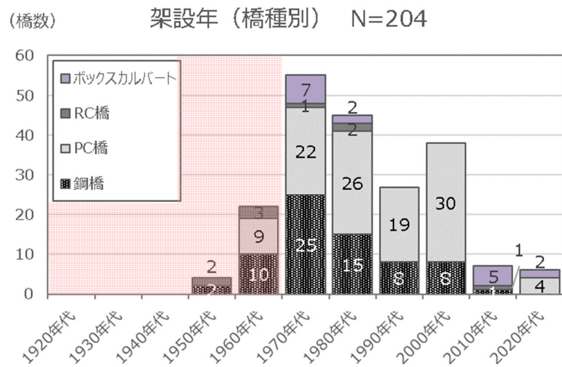
図 2.7 橋種別の架設年別橋梁数
