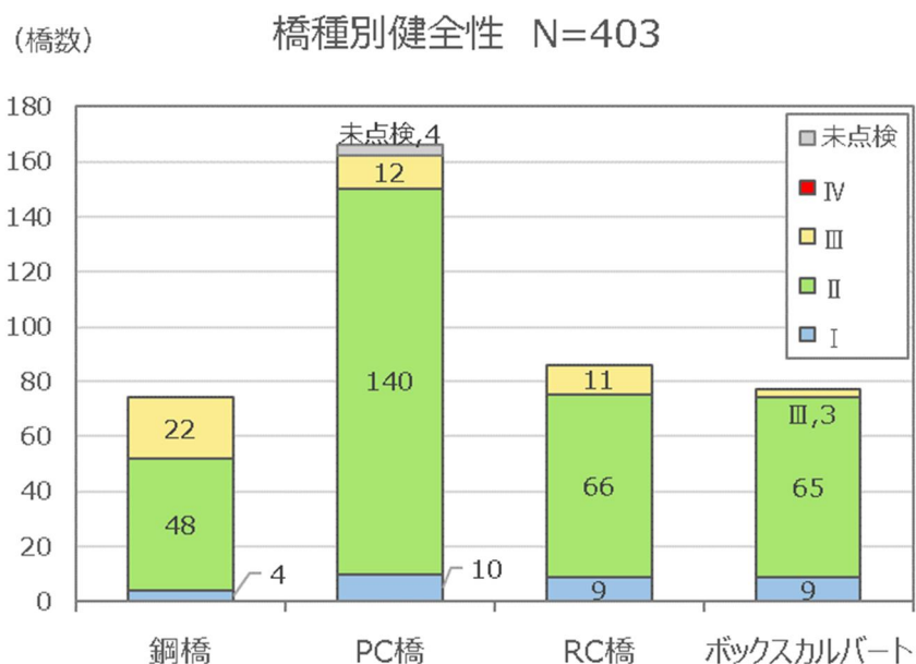
図 2.21 橋種別にみた橋梁の健全性
