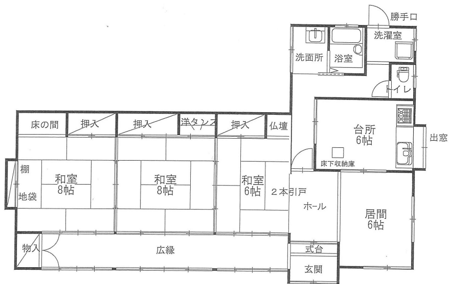
1階
